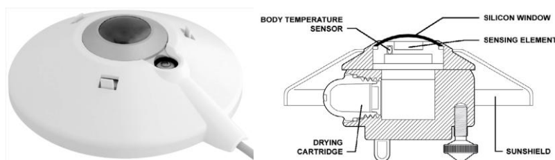
Figura 2: Pirgeômetro Kipp & Zonen Modelo CGR 4.
