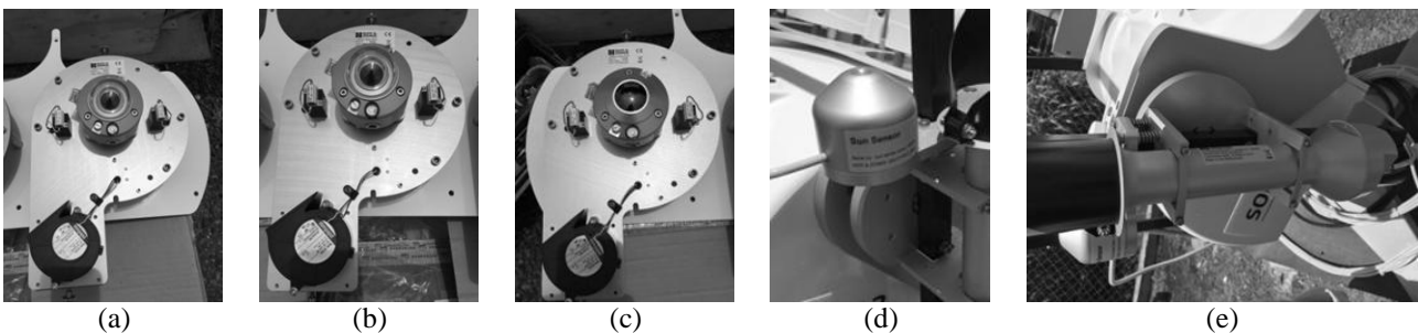
Figura 13: (a) Sensor Radiação Difusa, (b) Sensor Radiação Global, (c) Sensor Radiação Onda Longa, (d) Sun Sensor, (e) Sensor Radiação Direta.
