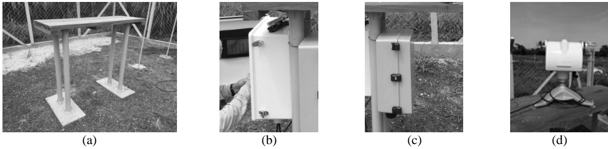
Figura 11: (a) Bancada, (b) caixa do datalogger , (c) caixa de passagem dos cabos, (d) Rastreador e sua base-tripé.
