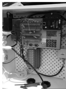
Figura 10: Caixa do datalogger .
