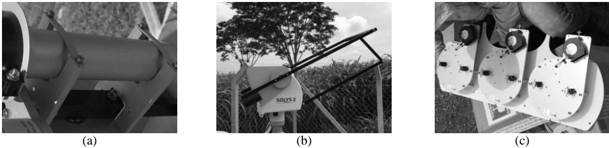
Figura 12: (a) Mira do rastreador, (b) Haste de sombreamento, (c) Mesa superior com unidades de ventilação.
