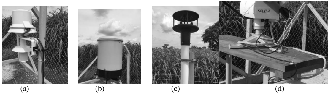
Figura 14: (a) TermoHigrômetro, (b) Pluviômetro, (c) Anemômetro 2D, (d) Cabeamento livre para movimento do rastreador.
