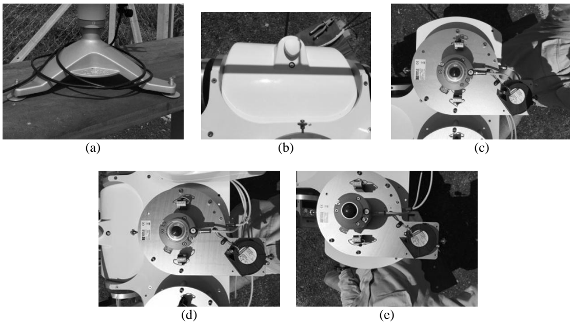
Figura 15: (a) Base-tripé, (b) Bolha de nivelamento do rastreador, (c) Sensor radiação difusa, (d) Sensor radiação global e (e) Sensor radiação onda longa.
