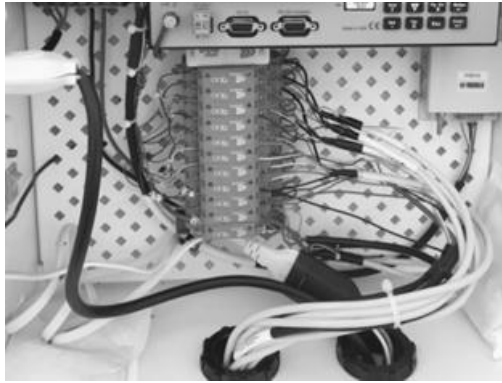
Figura 17: Ligação elétrica dos sensores ao datalogger .
