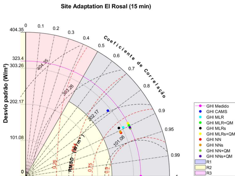
Figura 1 – Diagrama de Taylor para a divisão 1 dos dados (com randomização) da Estação Solarimétrica de El Rosal.
